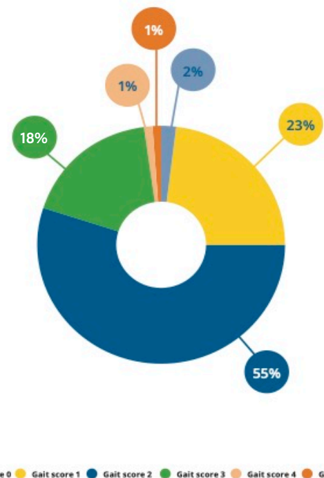
Gait score (0-5)
